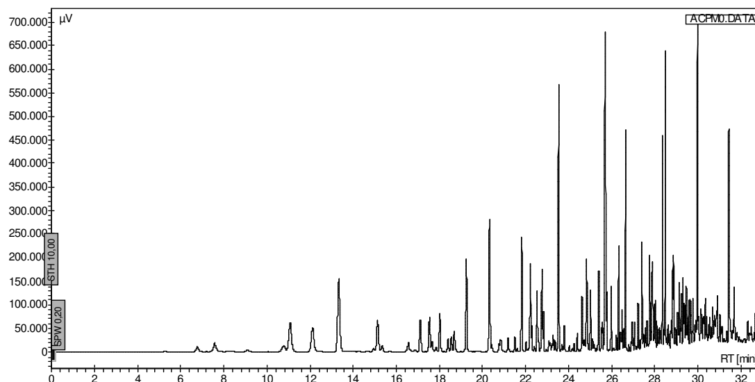
Figura 4. Perfil cromatográfico del ACPM.
