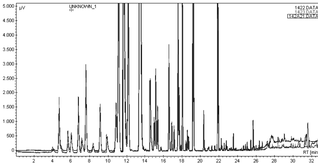
Figura 2. Triplicados de la muestra 142.
