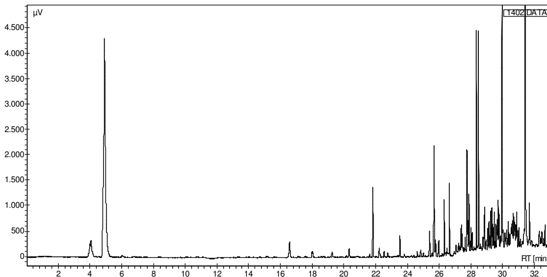
Figura 3. Perfil cromatográfico de la muestra 140.
